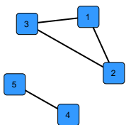
(b) G_{t=2}
