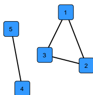
(b) G_{t=2}
