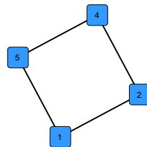
(c) G_{t=3}
