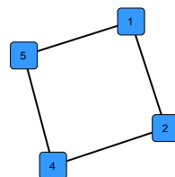
(c) G_{t=3}
