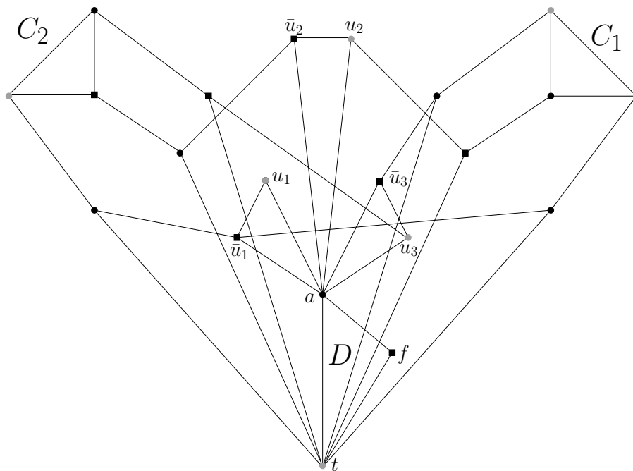
Abbildung 4.4: Graph zu einem 3SAT-Problem mit zwei Klauseln
