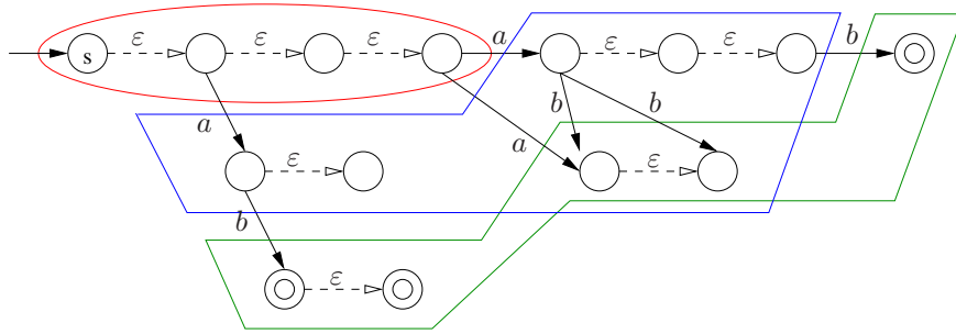
Abbildung 2.4: Mögliche Abarbeitungen von w = ab in einem NEA mit ab \in L , a \notin L
