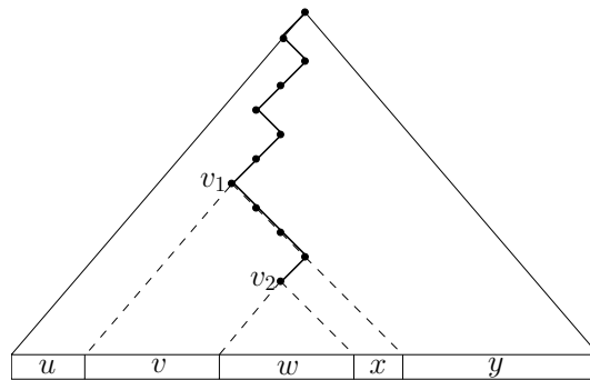
Abbildung 5.2: Weg im Syntaxbaum mit zwei Verzweigungsknoten v_1, v_2 , die derselben Variablen entsprechen.
