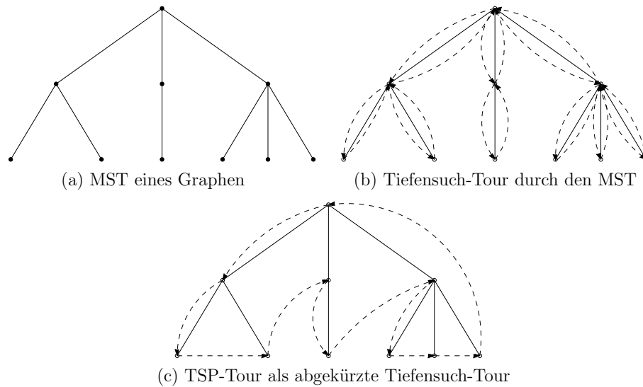
Abbildung 4.10: Konstruktion einer TSP-Tour mit Hilfe eines MST
