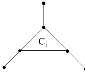
Abbildung 4.3: Komponente C_j
