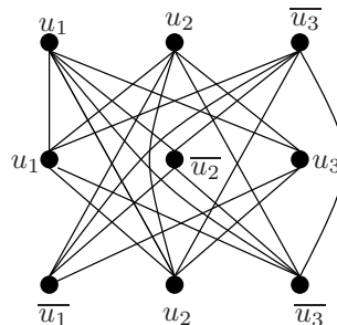
Abbildung 4.2: Graph G aus 3\text{SAT} \leq \text{CLIQUE}
