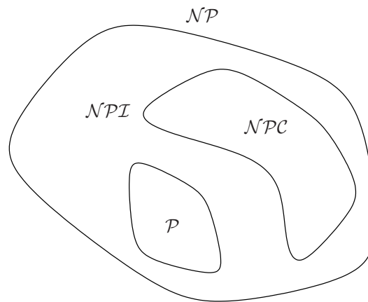
Abbildung 4.7: Komplexitätsklassen
