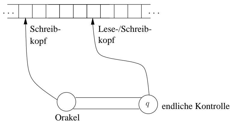
Abbildung 4.1: nichtdeterministische Turing-Maschine
