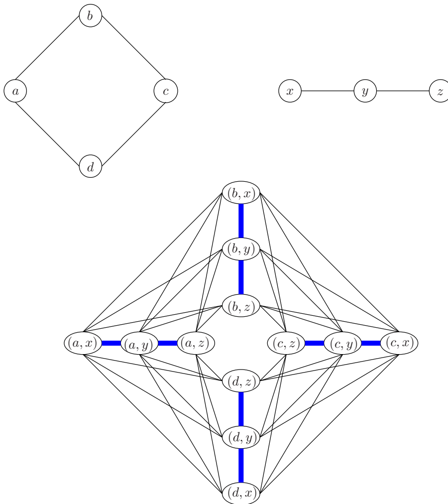
Abbildung 4.9: Graphen G_1 , G_2 und G_1[G_2] (von links nach rechts)
