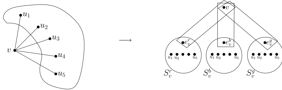
Abbildung 4.5: Konstruktion der Mengen S_v^c, c \in C , für einen Knoten v \in V eines Graphen G = (V, E) .
