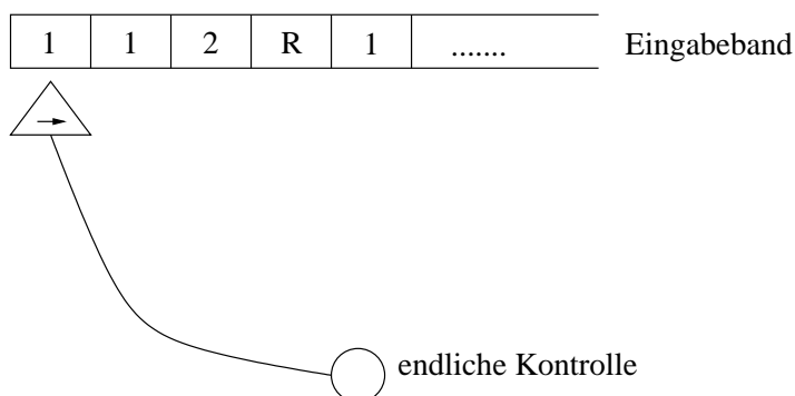
Abbildung 1.1: Modell für den Fahrkartenautomaten
