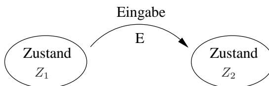
Abbildung 1.2: Zustandsübergang
