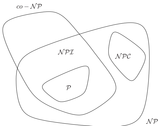
Abbildung 4.8: Komplexitätsklassen
