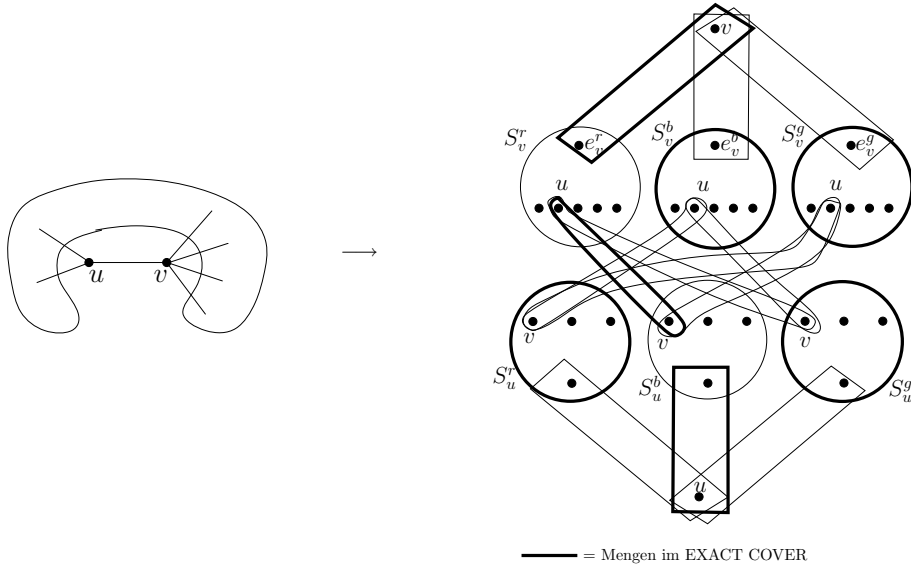
Abbildung 4.6: Konstruktion der Mengen \{u_v^c, v_u^{c'}\}, c \neq c' , für eine Kante \{u, v\} \in E eines Graphen G = (V, E) .
