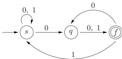
Abbildung 2.6: NEA für L
