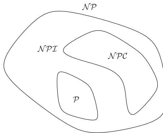
Abbildung 4.7: Komplexitätsklassen
