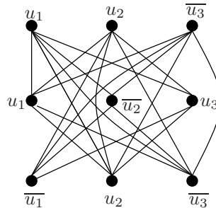
Abbildung 4.2: Graph G aus 3SAT \leq \mathcal{NP} CLIQUE
