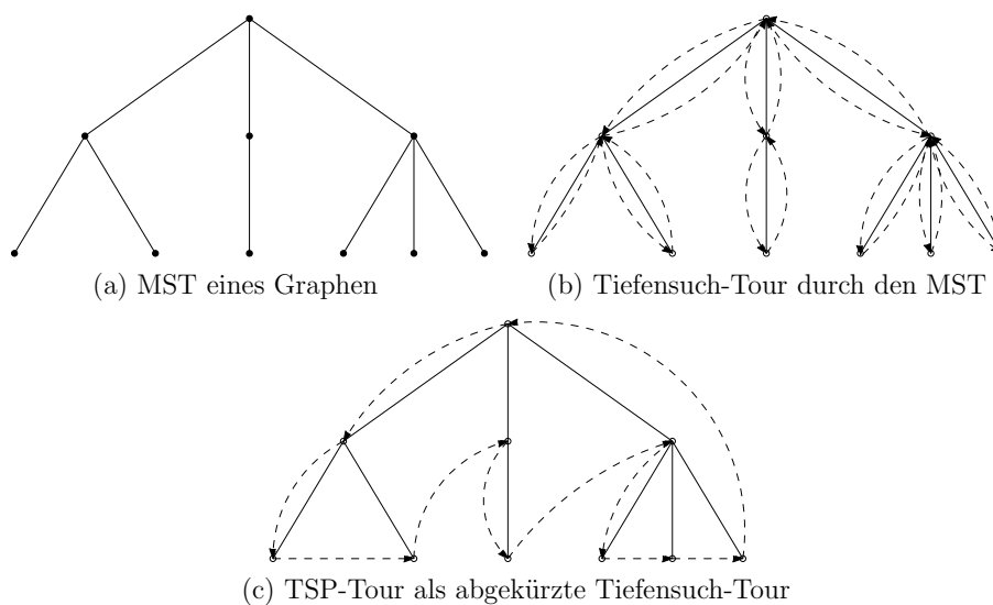
Abbildung 4.10: Konstruktion einer TSP-Tour mit Hilfe eines MST
