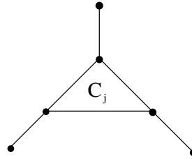
Abbildung 4.3: Komponente C_j
