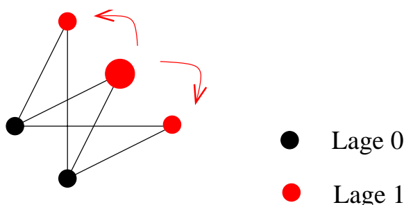
Abbildung 6.10: Festlegung der Lagen aller Konfliktsegmente eines Konflikt-Clusters durch Festlegung des Repräsentanten.
