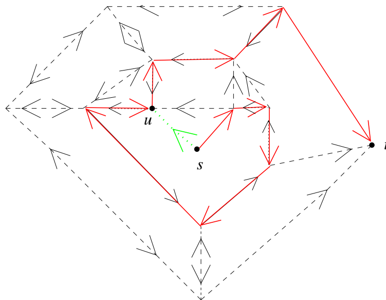
Abbildung 7.12: Die Situation nach dem ersten Suchschritt des zweiten Durchlaufes von 3. Der Suchweg (grün gestrichelt), d.h. s \rightarrow u trifft im Knoten u von rechts den s - t -Weg, der im ersten Durchlauf konstruiert wurde.
