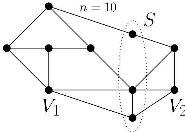
Abbildung 4.1: Ein Separator, der die Bedingungen des PLANAR-SEPARATOR-THEOREMS erfüllt.
