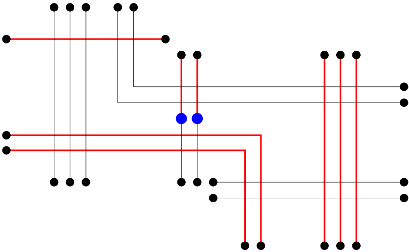
Abbildung 6.14: Realisierung des Layouts aus Abbildung 6.5 in zwei Lagen mit nur 2 Vias.
